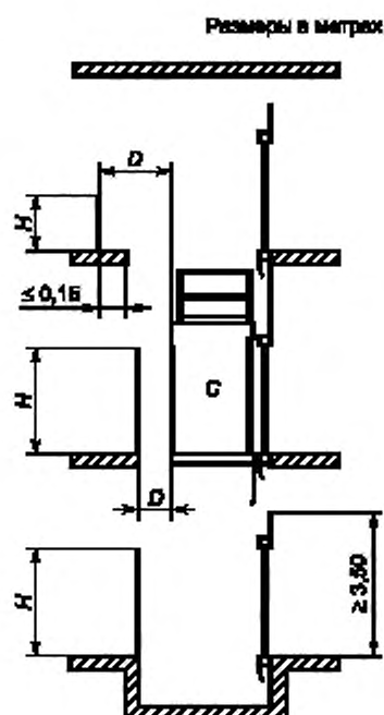
C — кабина; D — расстояние до движущихся частей лифта (см. рисунок 2); H — высота ограждения
